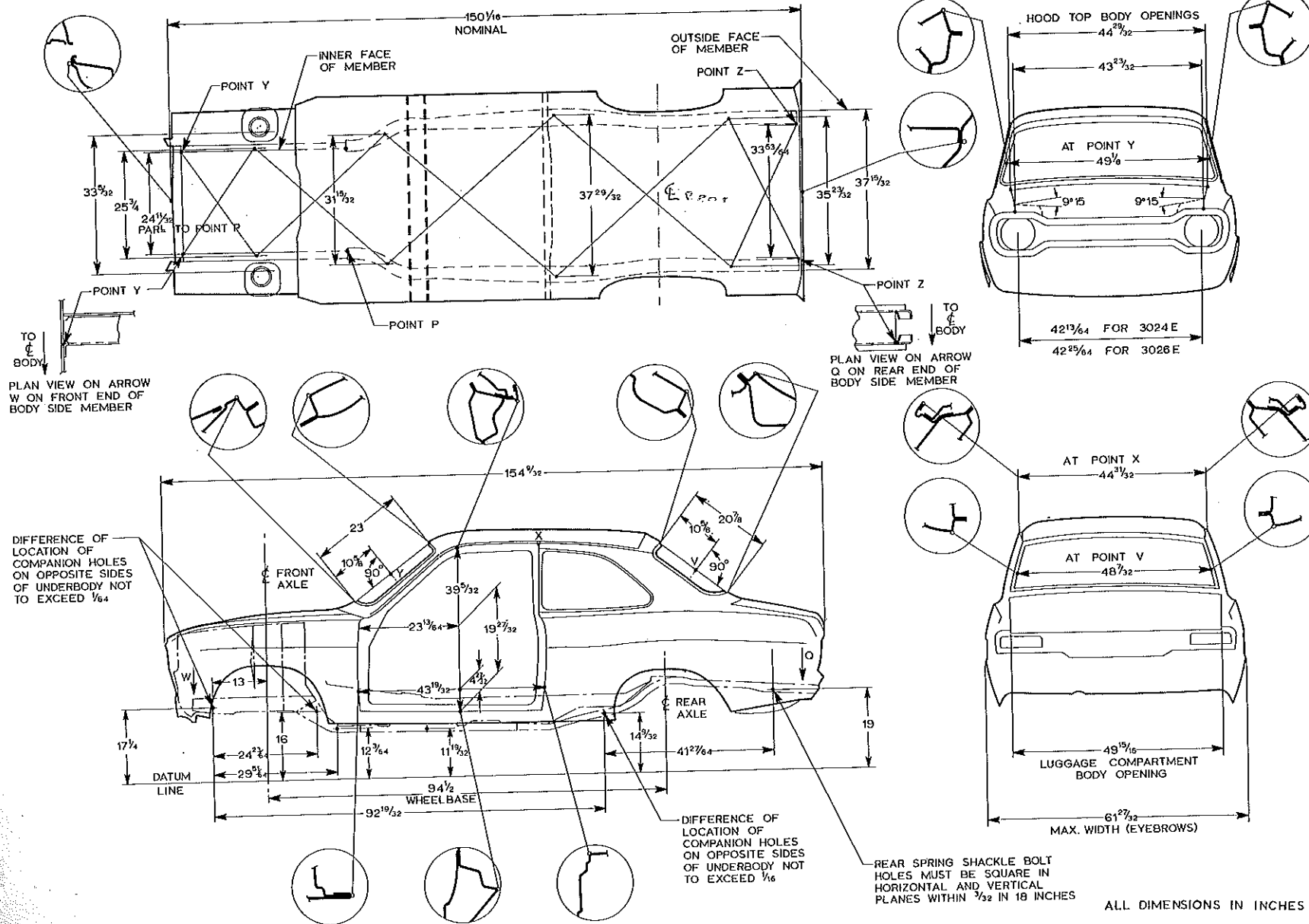
BODY TOLERANCE CHART (2 DOOR MODEL) SEDAN
